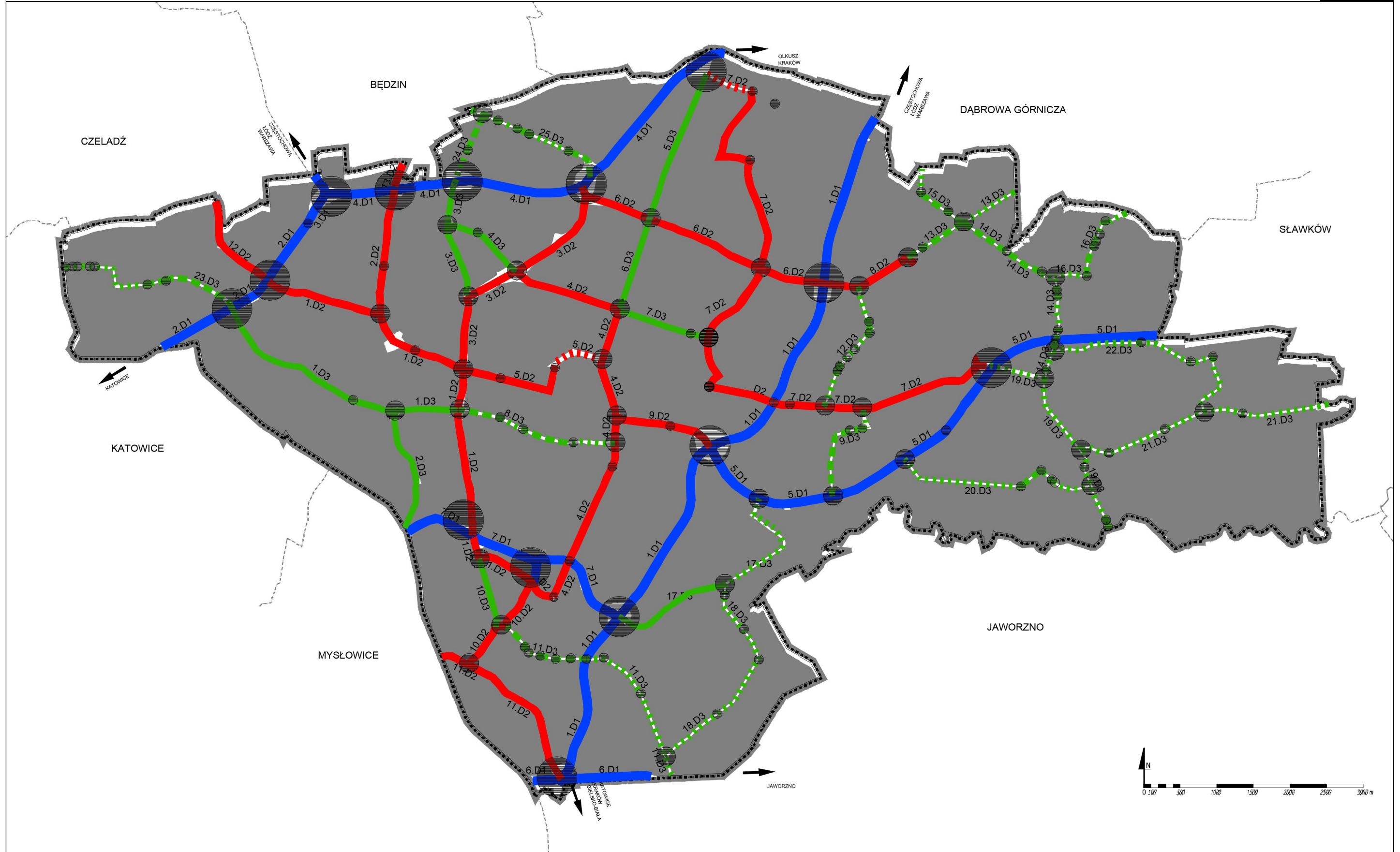
Rys. K/11 - Struktura Przestrzenna Stanu Docelowego - kierunki zmian układu drogowego, system dróg układów D1, D2, D3,
